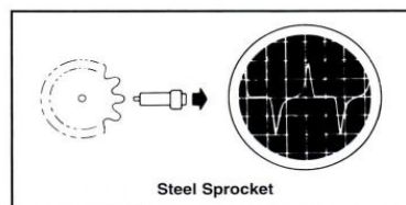
Steel Sprocket
